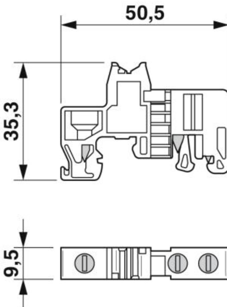
Dessin coté
