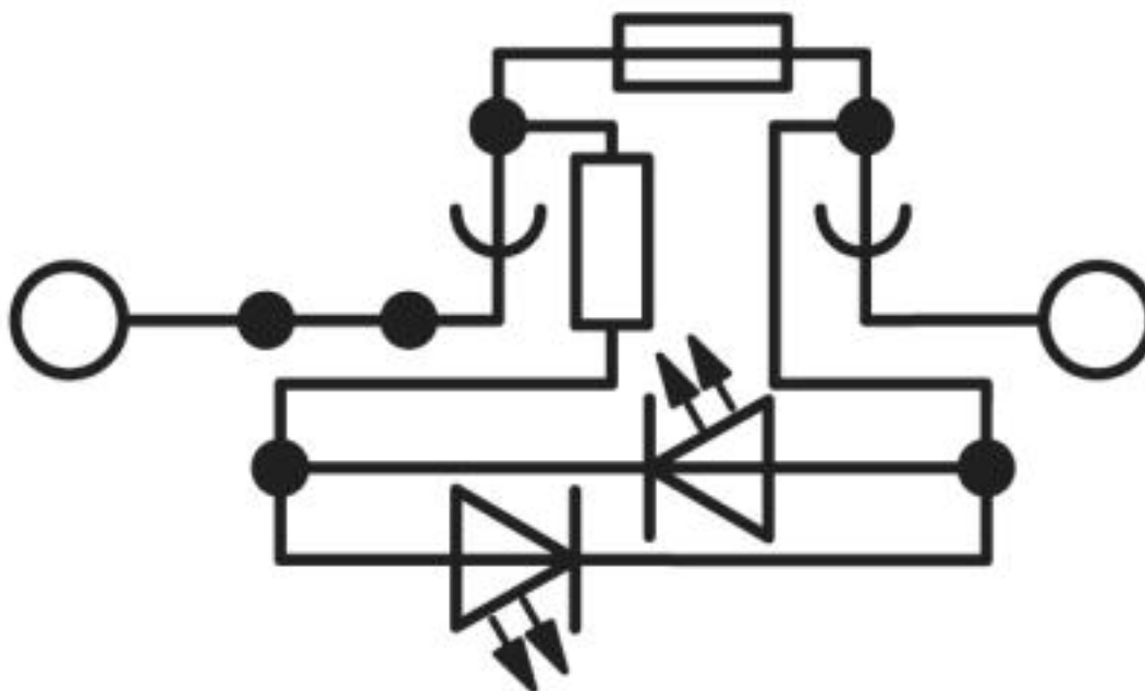
Diagrama eléctrico
