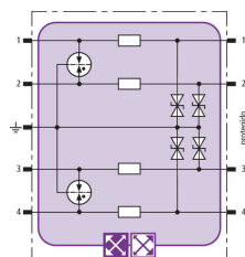
Esquema del BXT ML4 BE 180
