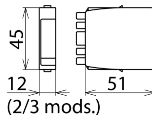
Dimensiones del BXT ML4 BE 180
