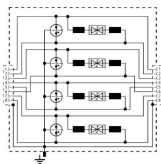
Esquema del DPA M CLE RJ45B 48
