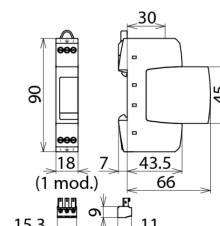
Dimensiones del DR M 2P 150 FM
