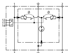
Esquema del DR M 2P 150 FM
